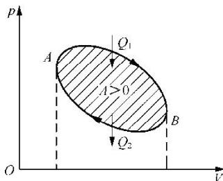
图 11-12 正循环
