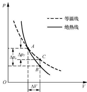
图 11-8 绝热线与等温线比较
