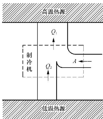
图 11-15 致冷机工作示意图
