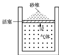
图 11-2 准静态过程
