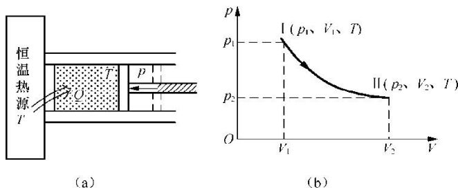
图 11-6 等温过程曲线
