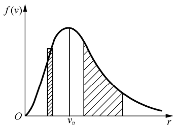
图 12-4 麦克斯韦速率分布曲线
