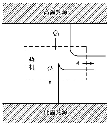
图 11-14 热机工作示意图
