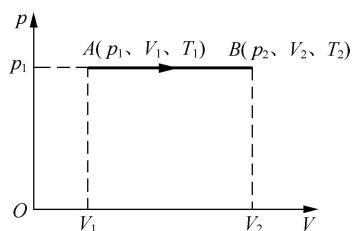
图 11-5 等压过程曲线
