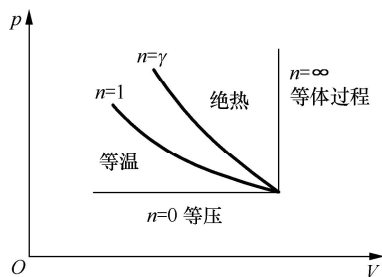
图 11-9 四种过程曲线
