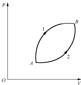
图 11-22 任意可逆循环
