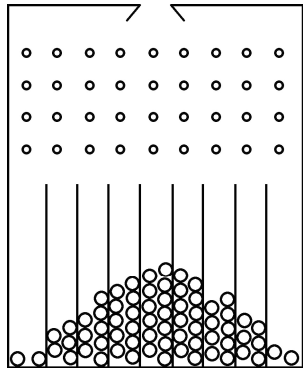
图 12-2 伽尔顿板实验
