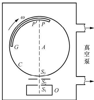
图 12-3 葛正权实验装置
