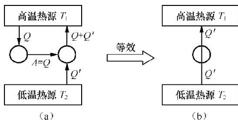
图 11-19 两个表述等价性证明之二
