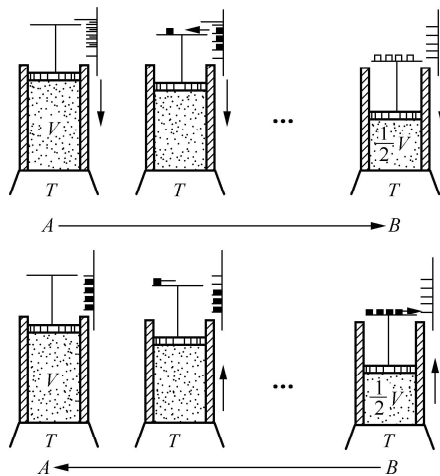
图 11-20 无摩擦的准静态过程
