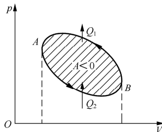
图 11-13 逆循环
