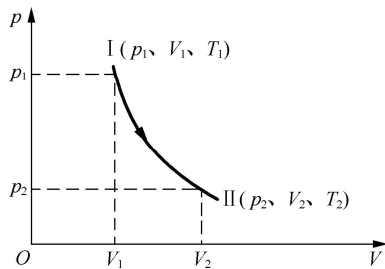
图 11-7 绝热过程曲线
