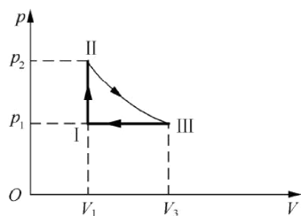
图 11-16 循环曲线
