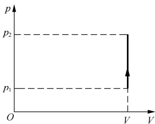
图 11-4 等体过程曲线
