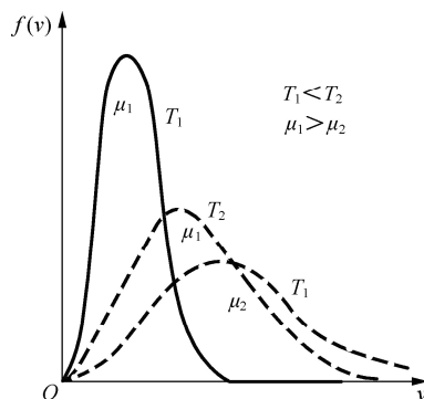
图 12-5 分子速率分布曲线与气体温度和分子质量的关系
