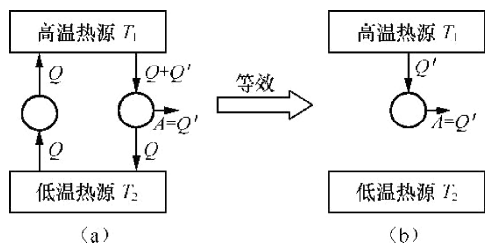
图 11-18 两种表述等价性证明之一
