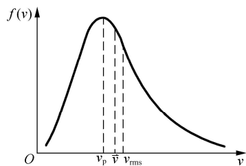
图 12-6 三种分子速率
