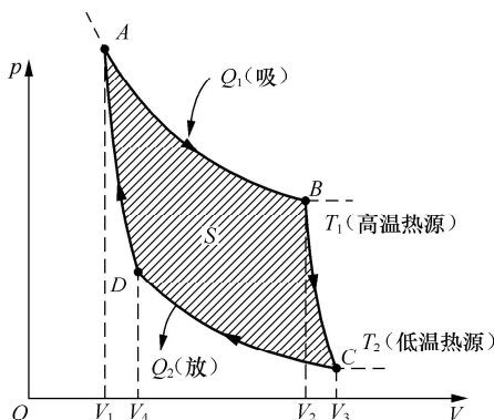
图 11-17 卡诺循环
