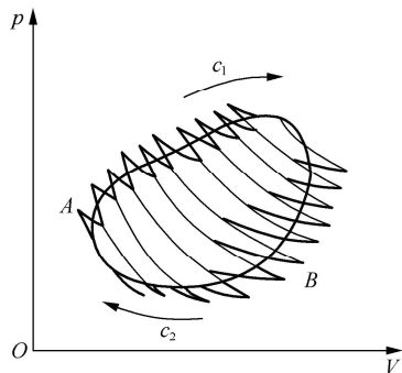
图 11-21 锯齿形曲线近似代替任意可逆循环过程
