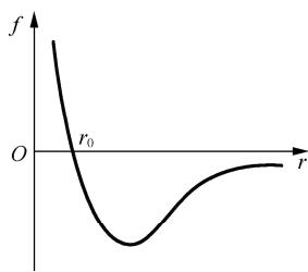
图 12-1 f(r) 与 r 的关系曲线
