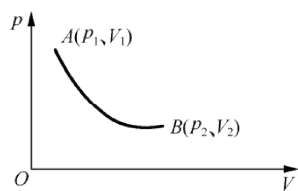
图 11-1 p-V 状态图
