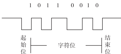
图 2-1 异步传输
