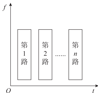
图 2-4 TDM 信道的划分
