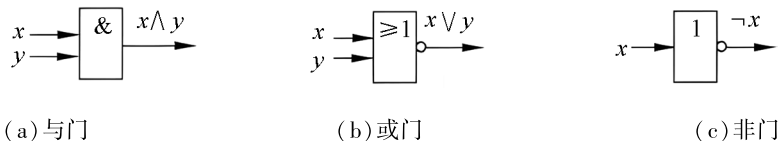
图 2.1 逻辑门
