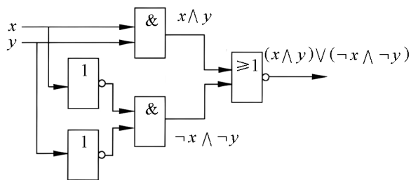
图 2.2 两个开关控制的灯具电路
